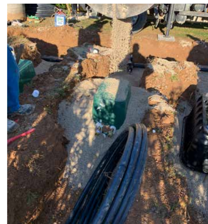
15 Les 10 derniers cm de la partie haute peuvent être remblayés avec la terre végétale
