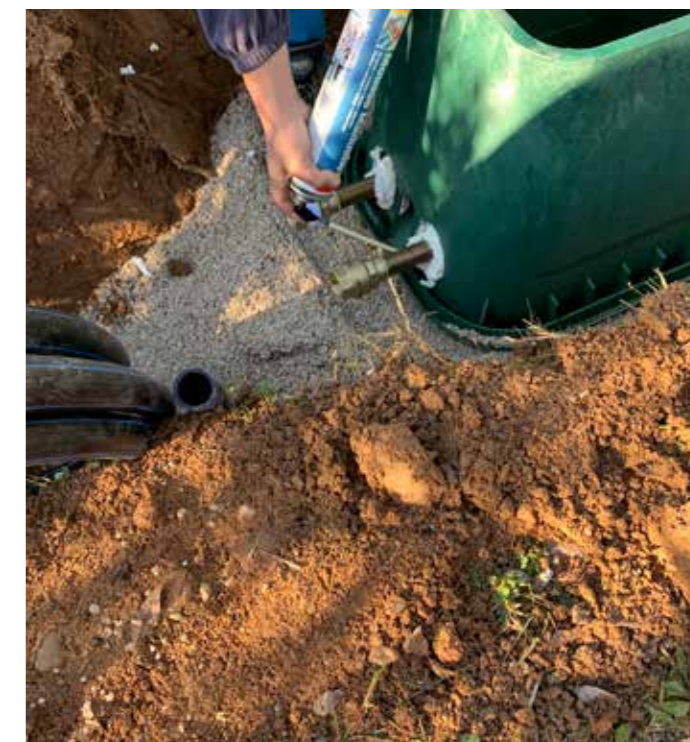
13 Etanchéification des entrées et sorties à la mousse PU
